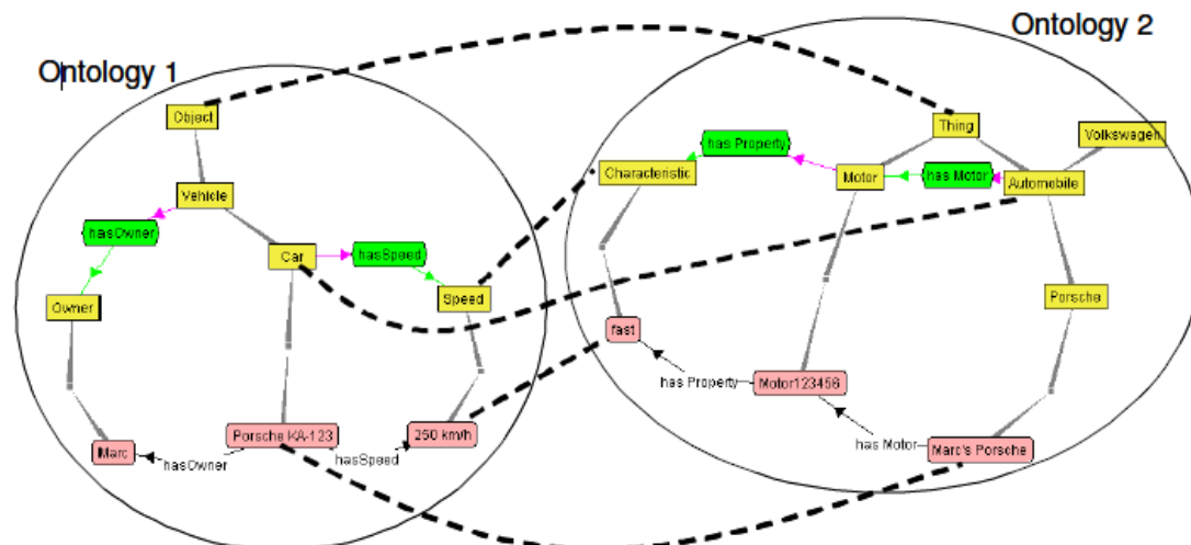
Εικόνα 8, Παράδειγμα Quick Ontology Mapping
