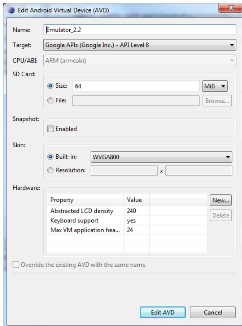
Εικόνα 22, Android emulator
