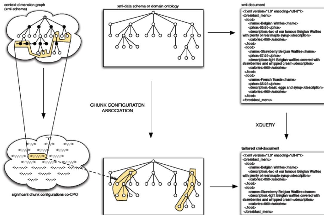
Εικόνα 6, Context Integrator
